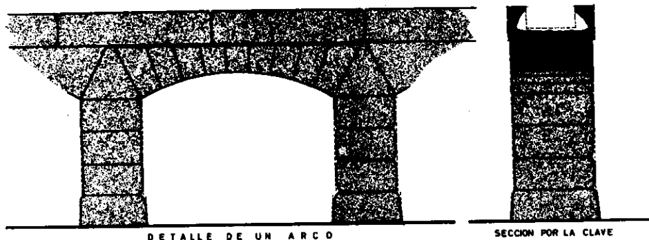
ACUEDUCTO ROMANO DE ALBATANA ESCALA EN METROS 0 0'25 0'50 0'75 1 1'25 1'50 2 ALBACETE MARZO 1973
